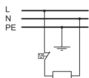
Überhitzungs- thermostat
