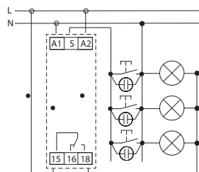
Anschluss von 3 Leitern
