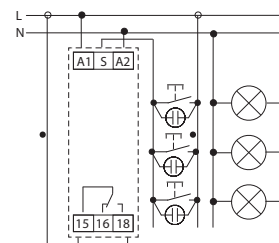
Anschluss von 4 Leitern
